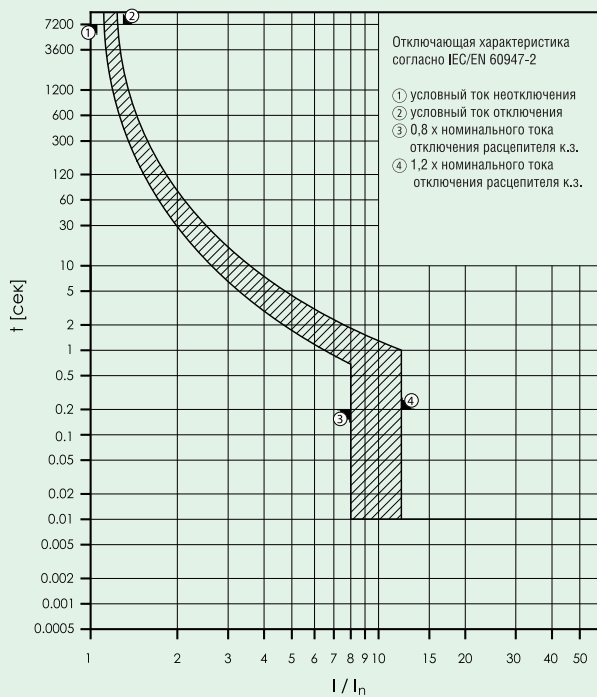
Кривая отключения VZM1 100A, 3-х полюсное исполнение
