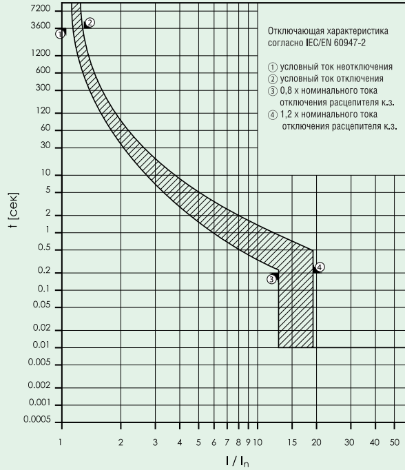
Кривая отключения BZM1 32A, 3-х полюсное исполнение
